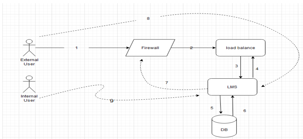
FIG.5. SOFTWARE SECURITY AT IUL
