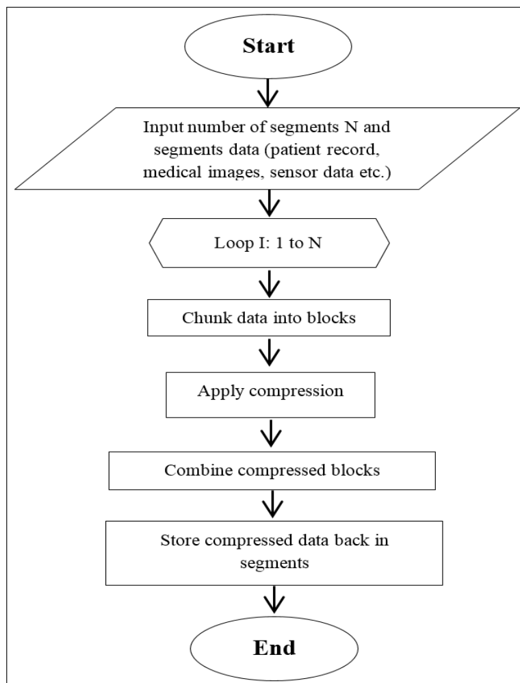
Fig. 6. SA steps.
