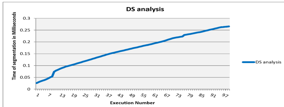
Fig. 14. DS evaluation.
